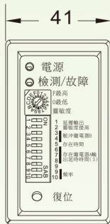
正視圖
